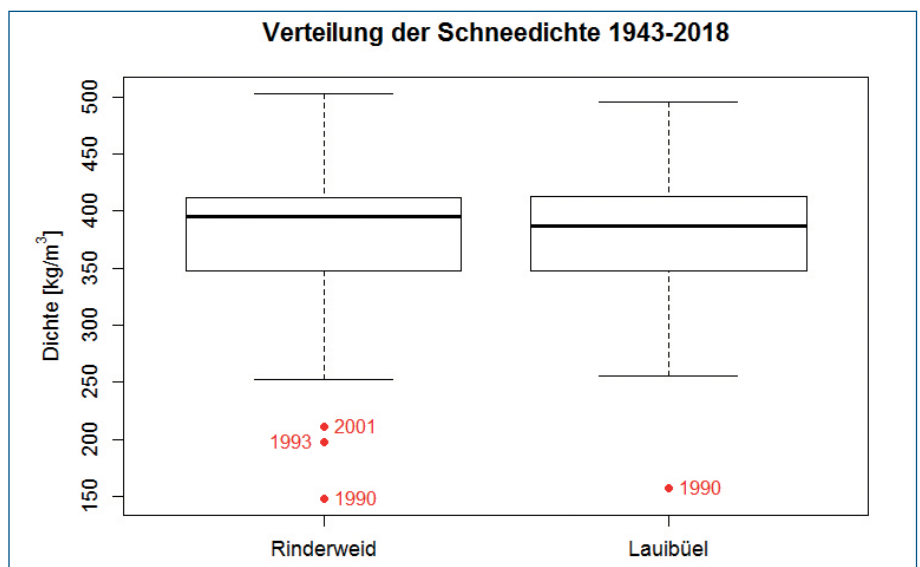
Bild 9. Box-Plot-Darstellung der ermittelten Schneedichten für die Messorte Rinderweid und Laubüel über die Messreihe 1943–2018 (jeweils am 1. April).
